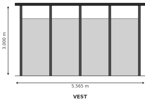
Figur 5. Snittegning, vest.
