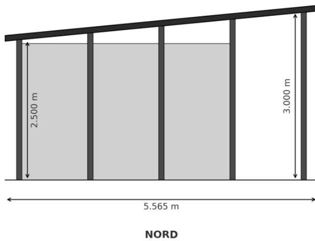
Figur 3. Snittegning, nord.
