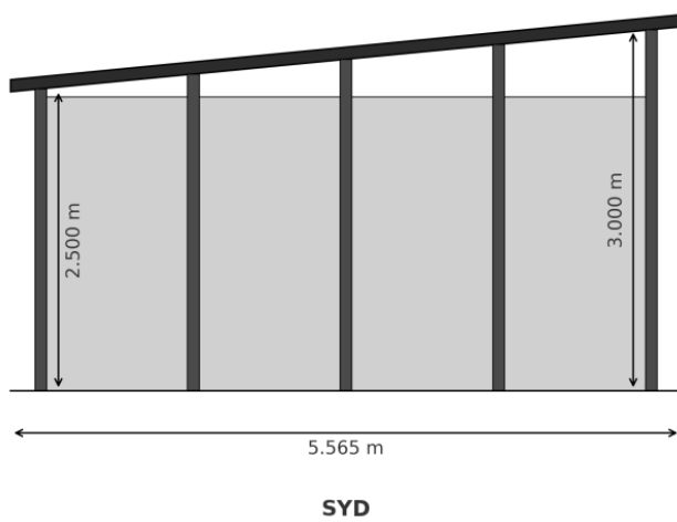
Figur 4. Snittegning, syd.
