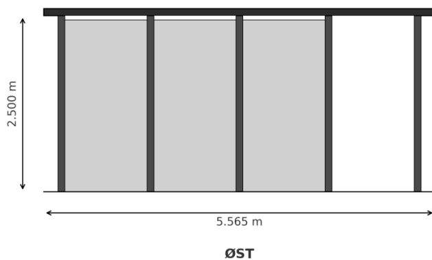
Figur 6. Snittegning, øst.
